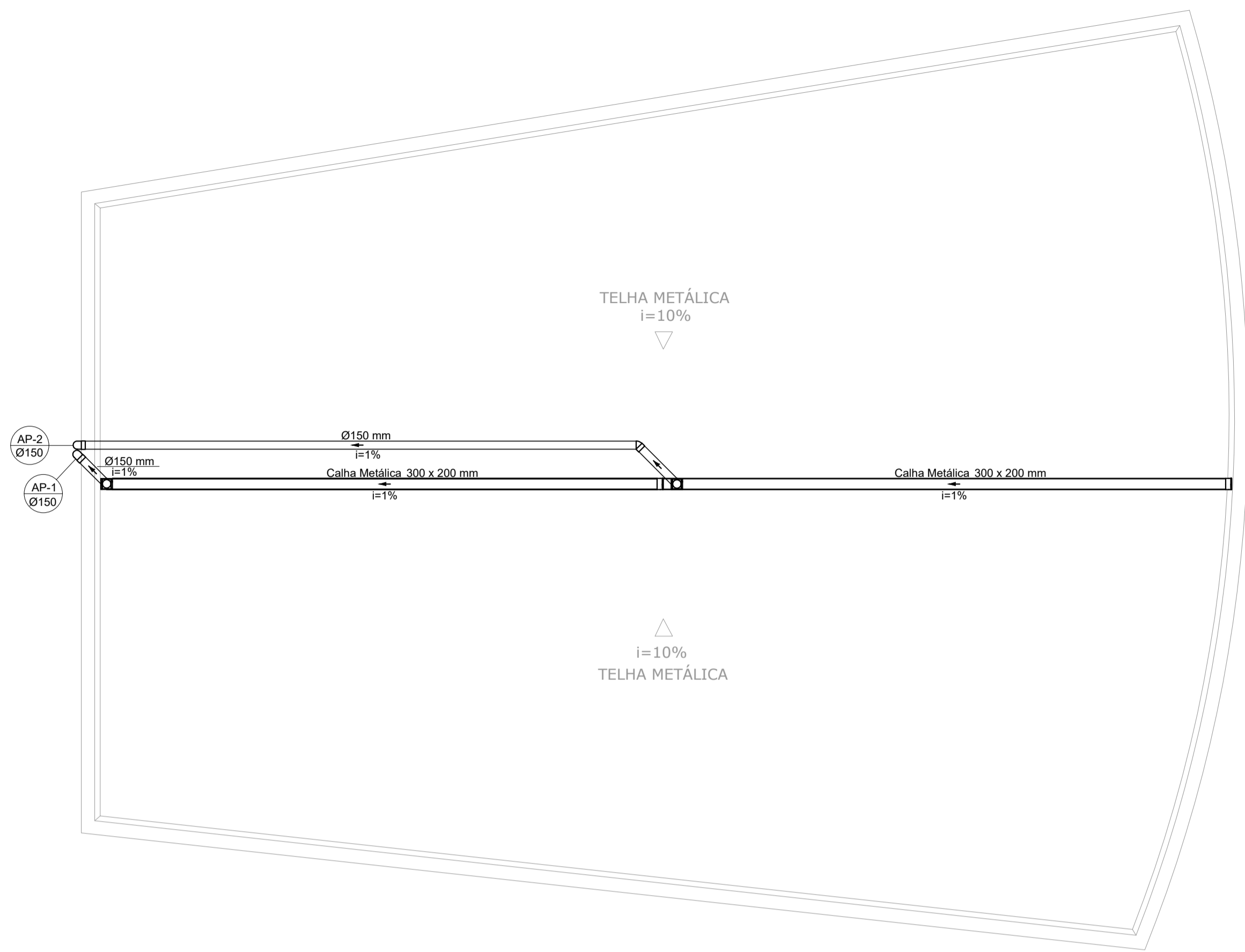
PLANTA BAIXA - COBERTURA ESCALA 1:75
