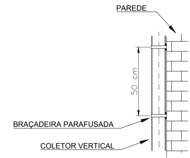
DETALHE A - FIXAÇÃO DO COLETOR VERTICAL
